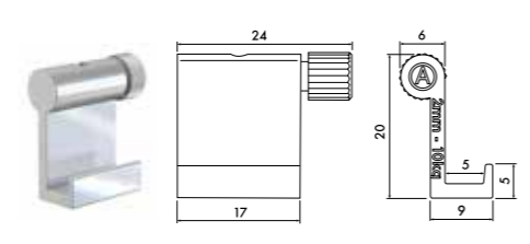
Auto Grip 10 kg
